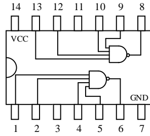
74LS20
