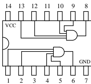
74LS21
