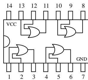
74LS32
