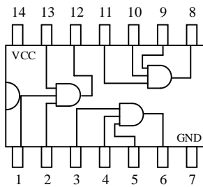
74LS15
