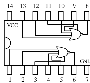
74LS25
