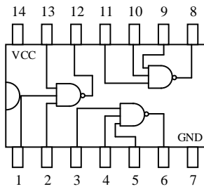
74LS12
