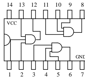
74LS11
