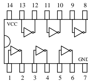
74LS16
