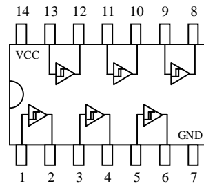
74LS14
