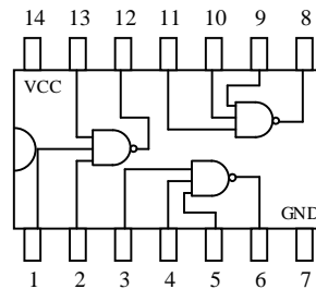
74LS10
