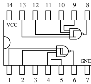
74LS13
