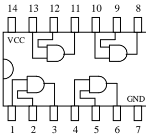
74LS09
