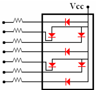
diagrama interno de um display de 7 segmentos anodo comum
